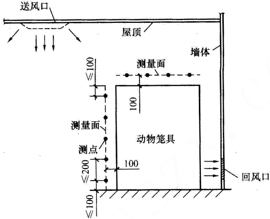
图 10.1.6 测点布置
