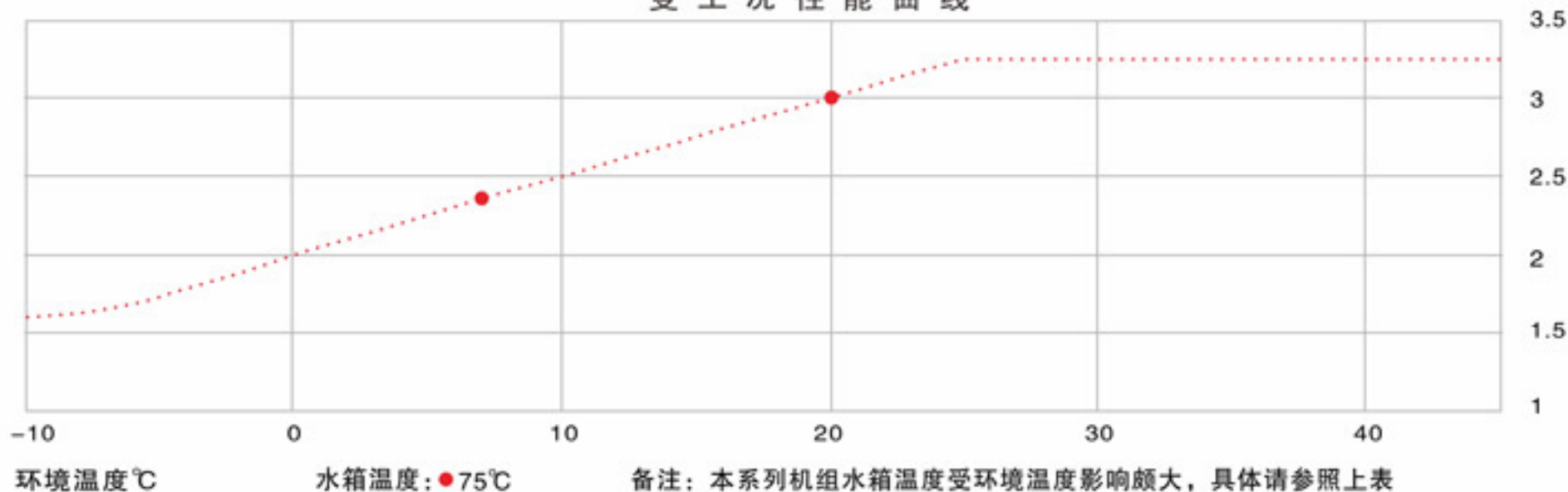
变工况性能曲线
