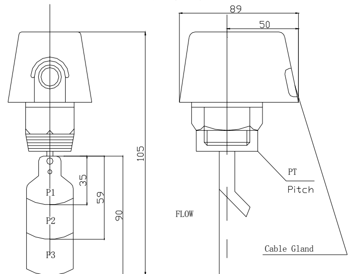
外形尺寸
