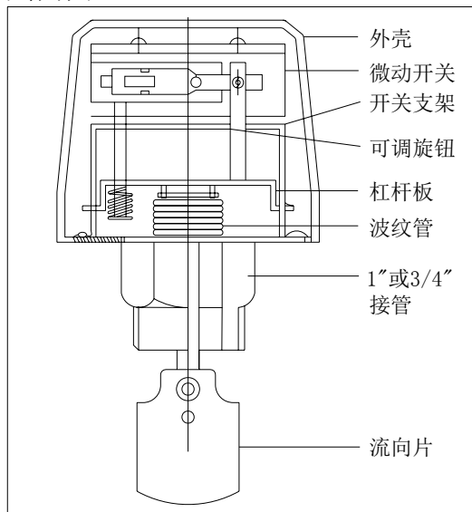
剖面图
