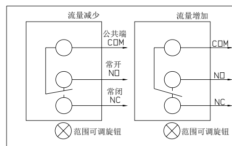
电气接线
