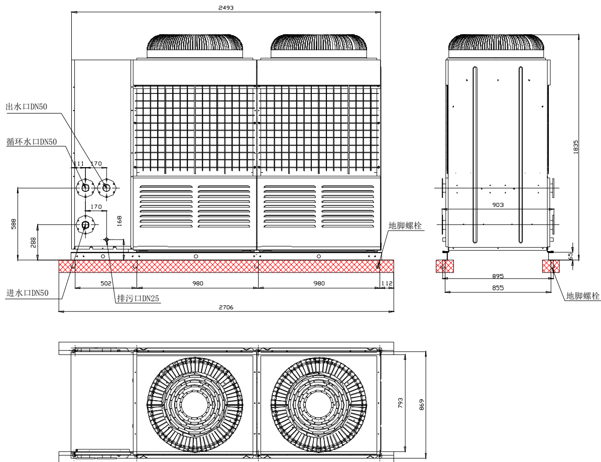
RSJ-770/S-820 外形图
