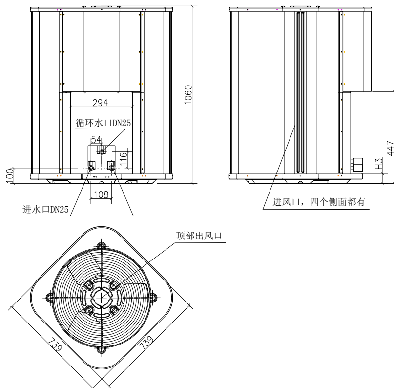
RSJ-200/S-540V、RSJ-100-540V 外形图
