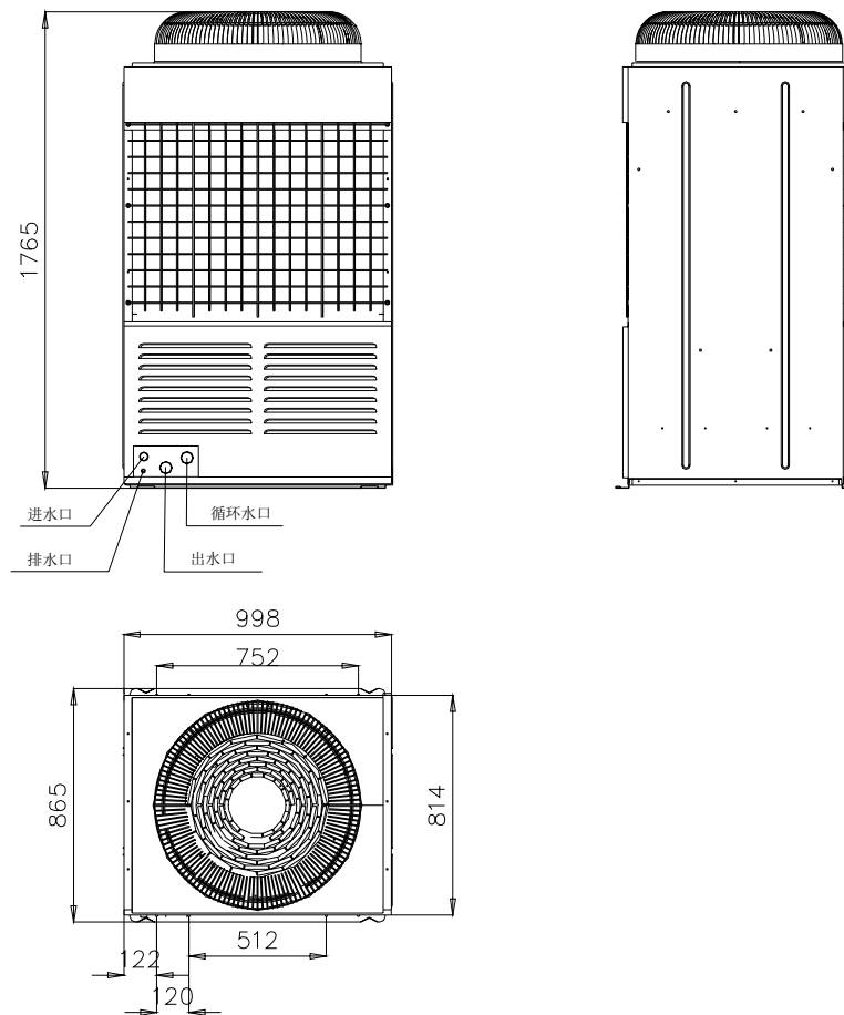
RSJ-200/S-540V、RSJ-100-540V 外形图
