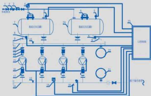
数字全变频双罐式无负压泵站系统图
