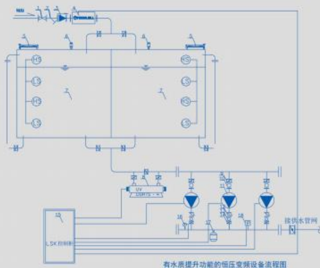
有水质提升功能的恒压变频设备流程图
