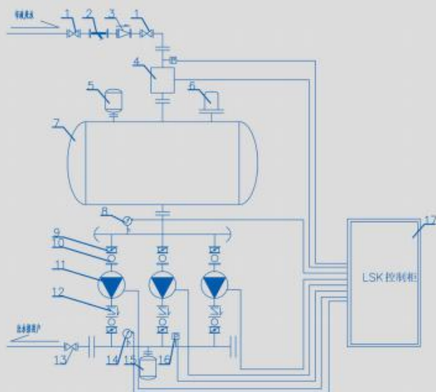
数字全变频稳压型罐式无负压设备系统图
